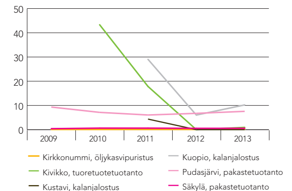
Sekajäte kg/tuotetonna 2009–2013
